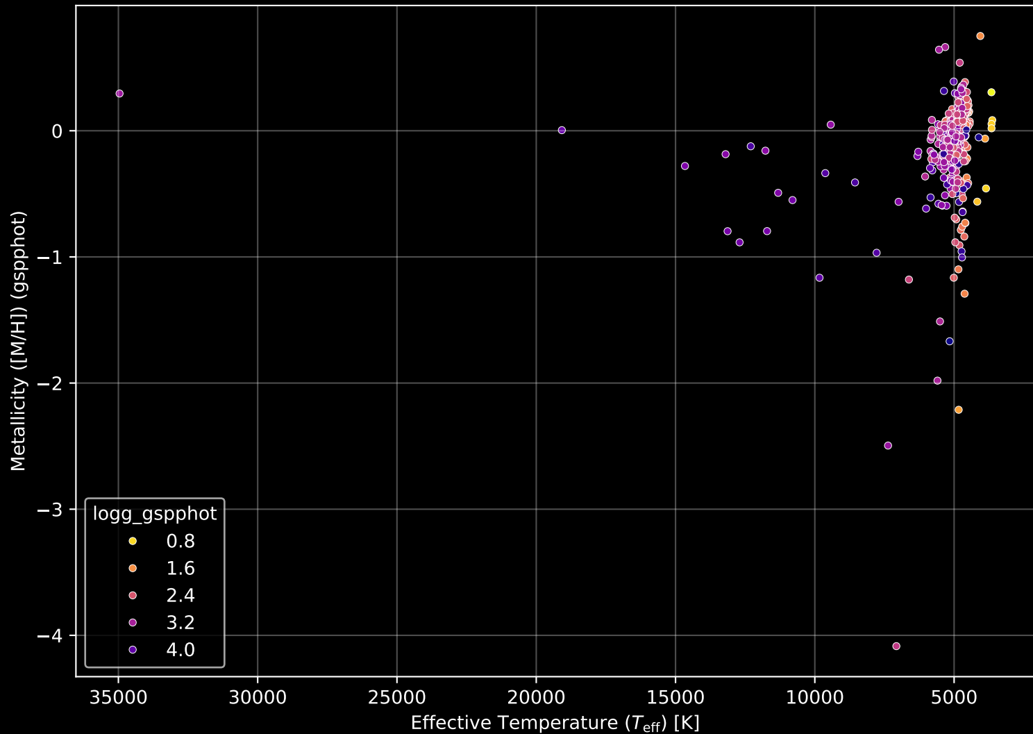
APOGEE DR17 Field: [030-08] Stellar Population Parameters (n= 568)
